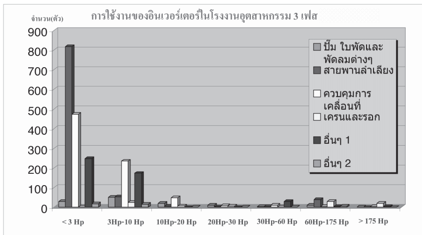
รูปที่ 2. การใช้งานอินเวอร์เตอร์ 3 เฟส ในโรงงานอุตสาหกรรม
